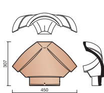
B000 5000 ① Rencontre 3D à emboîtement faîtière-arêtier 1/2 ronde Seltz
