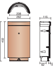
B000 1001 ① ② Faîtière-arêtier 1/2 ronde ventilée Seltz n°2 (90 cm 2 /ml) (2,5 au ml)
