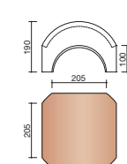
M000 5610 ① * Rencontre 4D base poinçon
