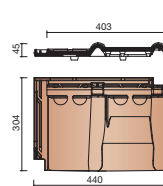
BOPA 8640 Tuile chatière (20 cm 2 ) (0,10 pc / m 2 projeté) ♦
