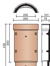
B000 1000 ① Faîtière-arêtier 1/2 ronde Seltz (2,5 au ml)
