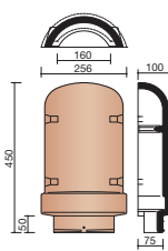
B000 1060 ① About arêtier 1/2 rond Seltz
