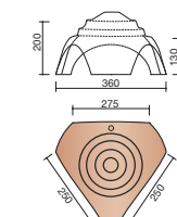
B000 5335 ① ② * Rencontre 3D base poinçon Élégante faîtières 1/2 rondes
