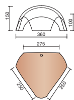
B000 5330 * Rencontre 3D base poinçon faîtières 1/2 rondes
