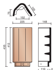
B000 2200 ① ② Faîtière d'abergement Shed (2,4 au ml)
