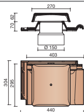
BOPA 8729 Kit tuile à douille Ø 150 mm (165 cm 2 )
